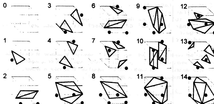
Figura 3.4: Los 15 patrones y su triangulación
