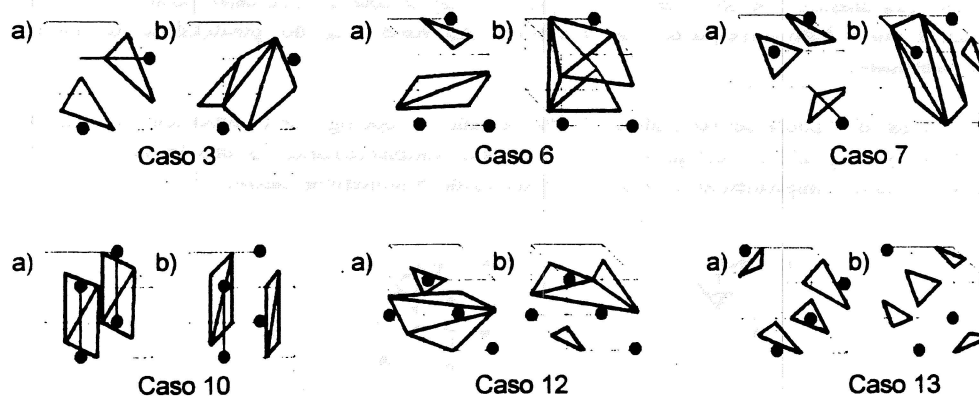
Figura 3.5: Los seis patrones ambiguos
