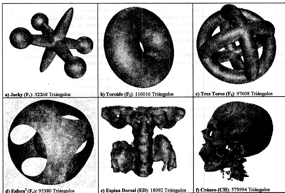
Figura 5.1: Imágenes resultantes de la triangulación
