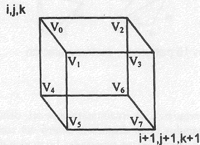
Figura 3.2: Los 8 vértices de un voxel
