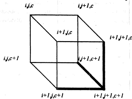
Figura 4.1: Aristas asociadas a IV[c,i,j]
